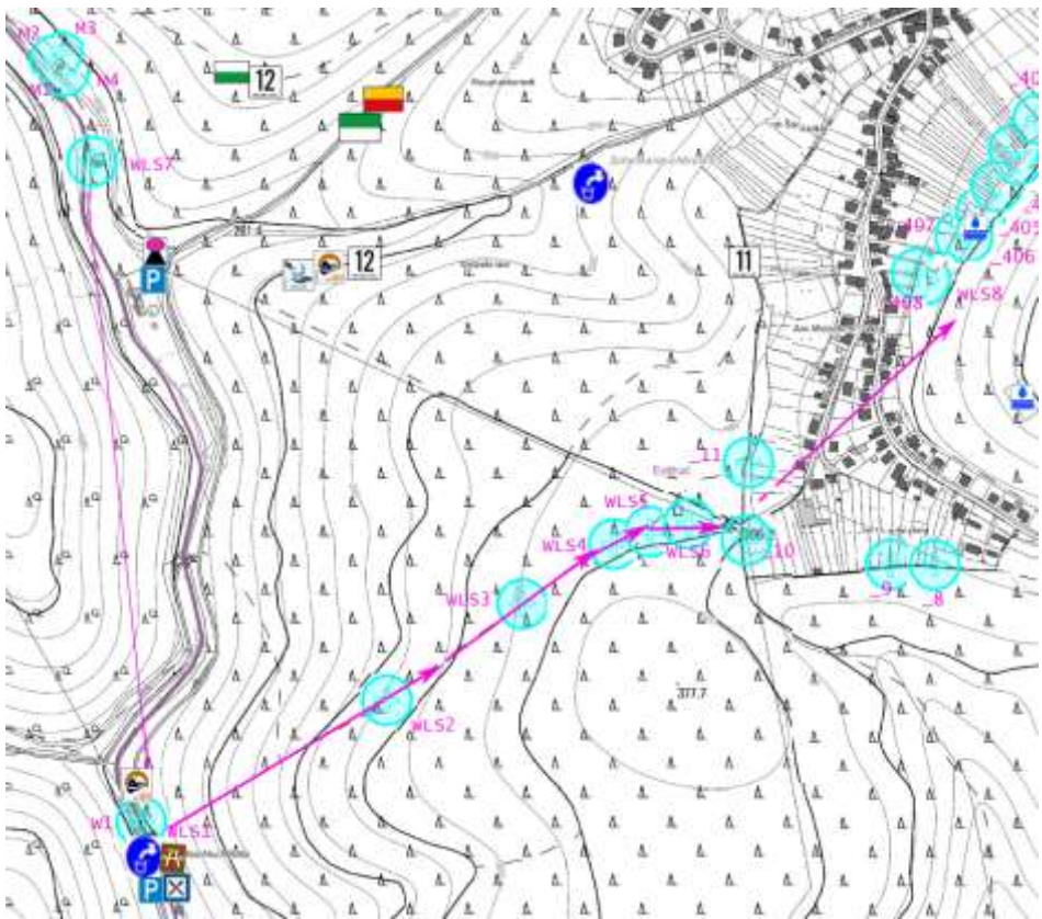
Verlauf der Trinkwasserleitung vom Mühlbrunnen - Wolfsschluchthütte hoch nach Esthal
